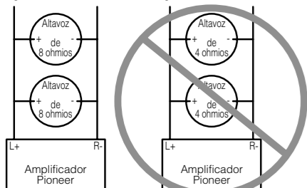
Modo de conexión en puente de 4 ohmios Modo de conexión en puente de 2 ohmios
