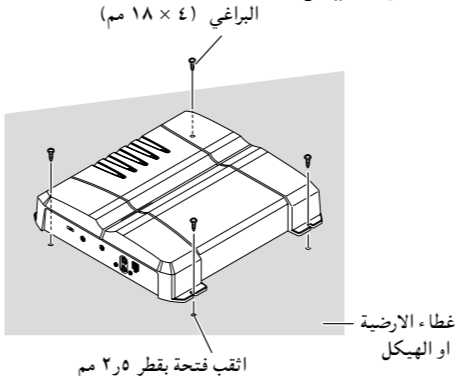
اثقب فتحة بقطر ٢.٥ مم
