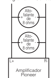
Modo de conexão em ponte de 4 ohms
